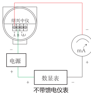
两线制4~20mA接线图二
